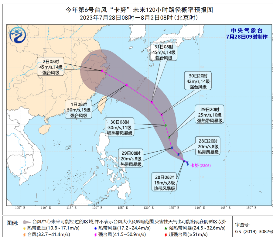
图 2 台风“卡努”路径最新预报图
