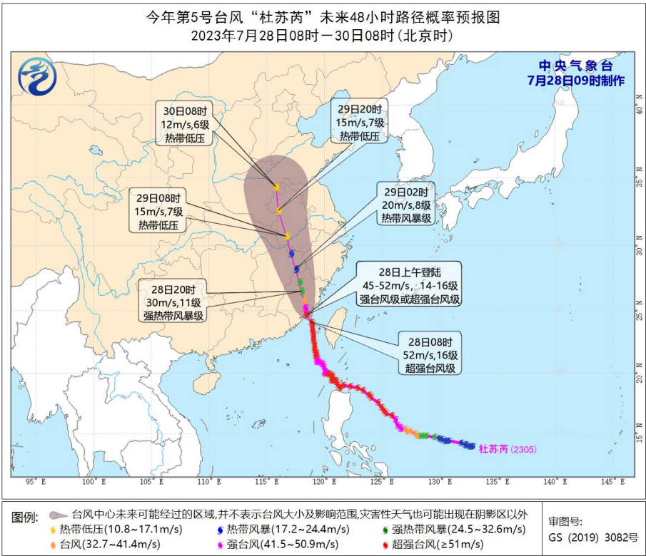
图 1 台风“杜苏芮”路径最新预报图
