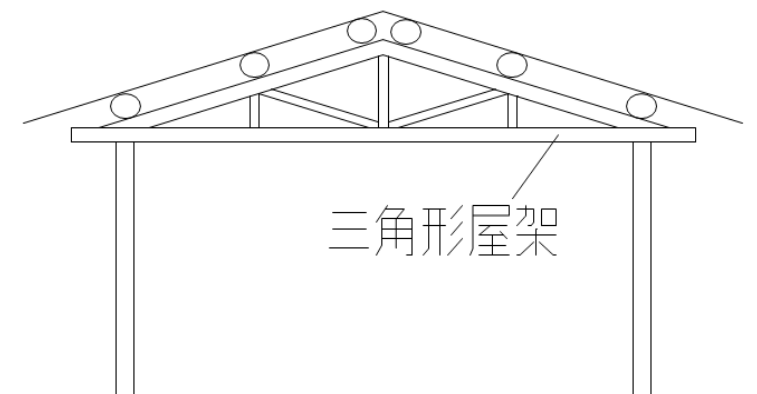
木屋架
