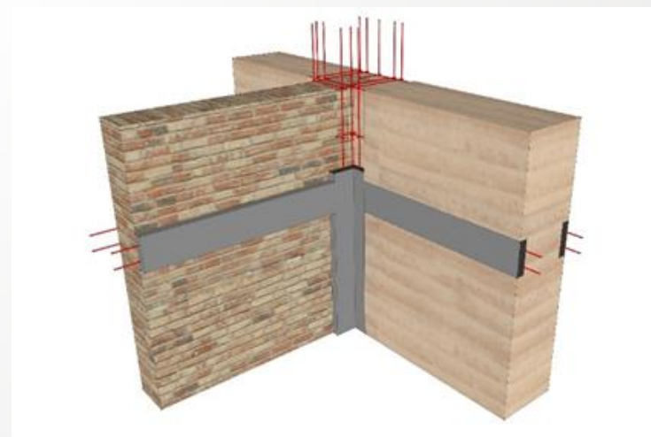
配筋砂浆带加固节点示意
