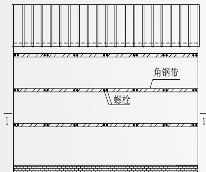
(a) 墙体正立面图
